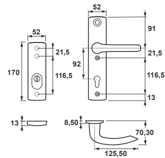
Solo Jupiter Electro Flex Premium Klamka+Krótki szyld, rozstaw 92 mm
