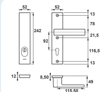
Solo Royal++ Flex Klamka+Długi szyld, rozstaw 92 mm
