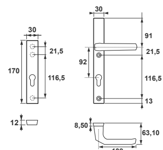
Solo Slim++ Klamka+Krótki szyld, rozstaw 92 mm
