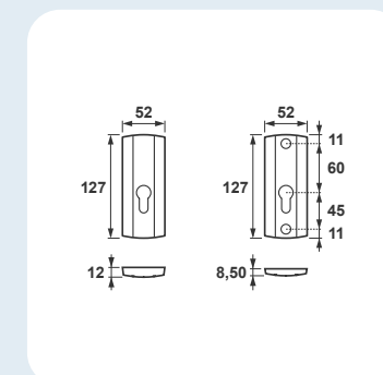
Prestige++ Rozeta długa
