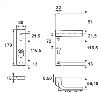
Solo Solid Flex Premium Klamka+Krótki szyld, rozstaw 72 mm
