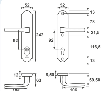
Verona++ Flex Klamko-klamka, rozstaw 92 mm
