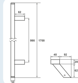
Amsterdam Skos 170 cm
