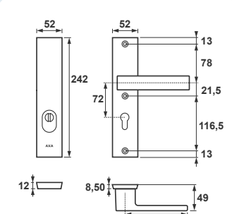
Solo Royal++ Flex Klamka+Długi szyld, rozstaw 72 mm
