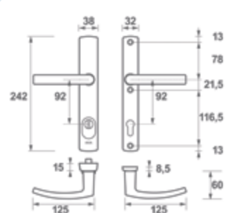
Narrow Klamko-klamka, rozstaw 92 mm
