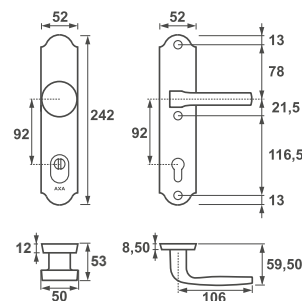
Verona++ Flex Klamko-gałka, rozstaw 92 mm
