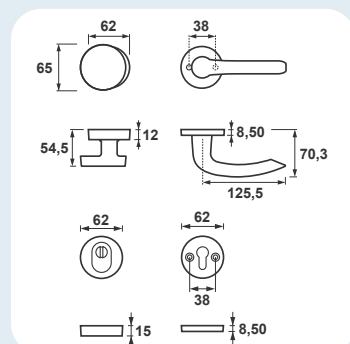
Diana Flex Click Klamko-pochwyt
