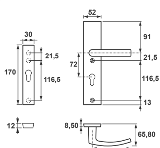
Solo Gaja++ Klamka+Krótki szyld, rozstaw 72 mm
