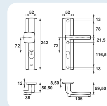
Prestige++ Flex Klamko-gałka, rozstaw 72 mm
