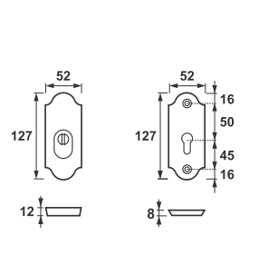
Solo Verona++ Flex Rozeta
