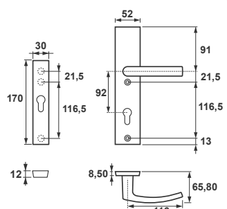
Solo Gaja++ Klamka+Krótki szyld, rozstaw 92 mm
