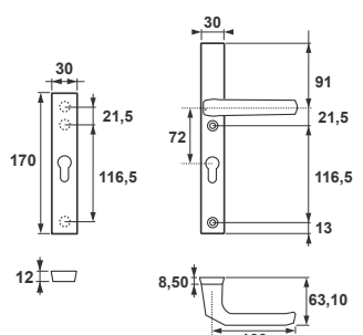
Solo Slim++ Klamka+Krótki szyld, rozstaw 72 mm
