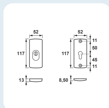
Solid Flex Premium Klamko-pochwył, rozstaw 92 mm
