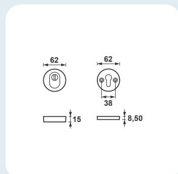
Diana Flex Click Rozeta
