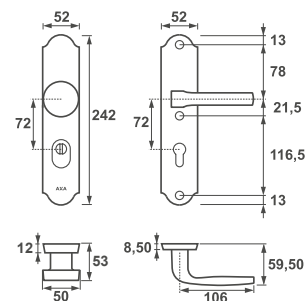
Verona++ Flex Klamko-gałka, rozstaw 72 mm
