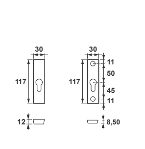
Solo Slim++ Rozeta
