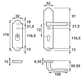
Solo Verona++ Flex Klamka+Krótki szyld, rozstaw 72 mm
