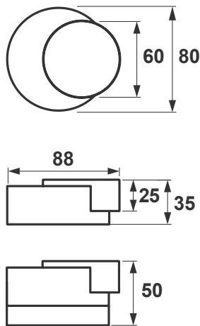
Odbojnik z modułem 15 mm
