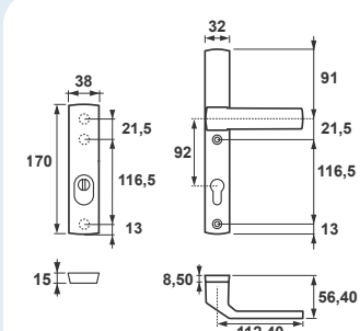
Solo Solid Flex Premium Klamka+Krótki szyld, rozstaw 92 mm
