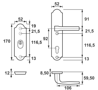
Solo Verona++ Flex Klamka+Krótki szyld, rozstaw 92 mm
