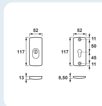
Jupiter Flex Premium Klamko-klamka, rozstaw 92 mm
