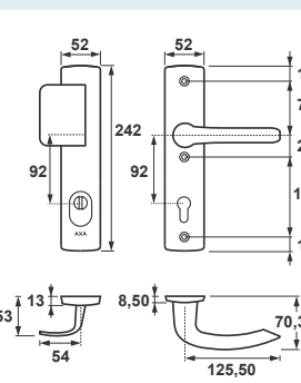
Jupiter Flex Premium Klamko-pochwyt, rozstaw 92 mm
