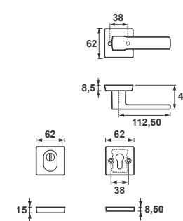
Solo Solid Flex Premium Klamka+Krótki szyld, rozstaw 92 mm
