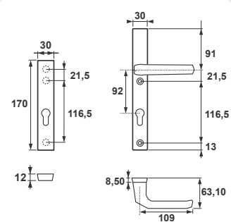
Solo Slim++ Klamka+Krótki szyld, rozstaw 92 mm
