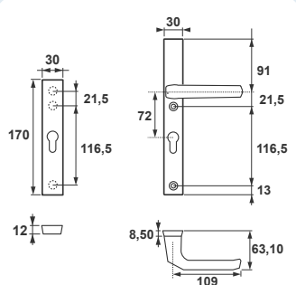
Solo Slim++ Klamka+Krótki szyld, rozstaw 72 mm
