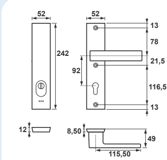
Solo Royal++ Flex Klamka+Długi szyld, rozstaw 92 mm
