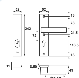
Solo Royal++ Flex Klamka+Długi szyld, rozstaw 72 mm
