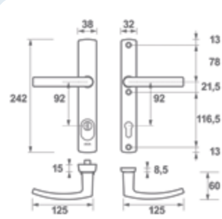
Narrow Klamko-klamka, rozstaw 92 mm
