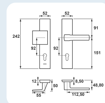
Leonardo Premium Click Klamko-pochwyt, rozstaw 92 mm
