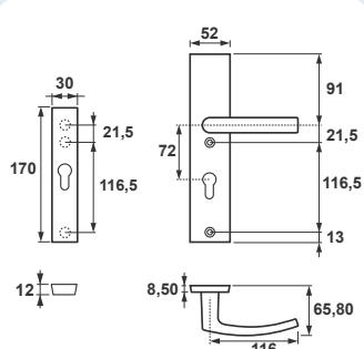
Solo Gaja++ Klamka+Krótki szyld, rozstaw 72 mm
