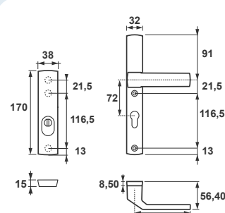
Solo Solid Flex Premium Klamka+Krótki szyld, rozstaw 72 mm
