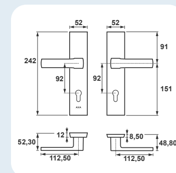
Leonardo Premium Click Klamko-pochwyt, rozstaw 92 mm
