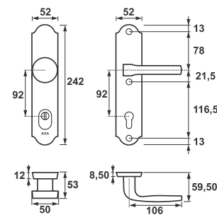
Verona++ Flex Klamko-gałka, rozstaw 92 mm
